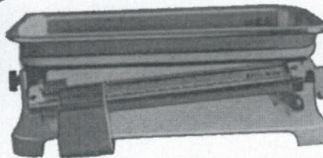
Laufgewicht- Haushaltswaage
