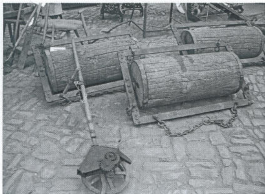
Holzwalzen zum Glätten des Saatbeetes und im Vordergrund ein Särab zum Ausbringen von Saatgut auf kleinen Flächen.
