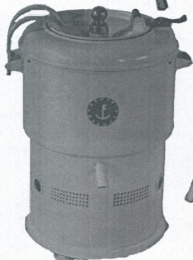
Trocken-Schleuder „Zentri-Krauß“
