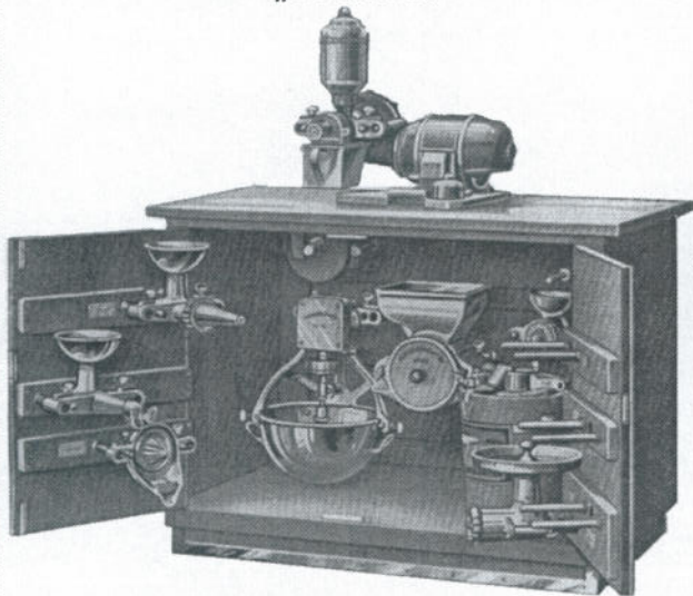
Elektrisch betriebene „Alexandertwerk-Küchenmaschine“
