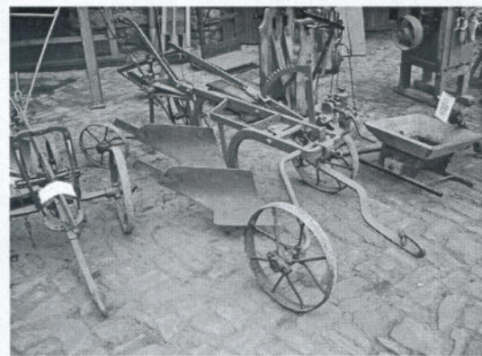
Pferdepflüge und Pflugscharren.
