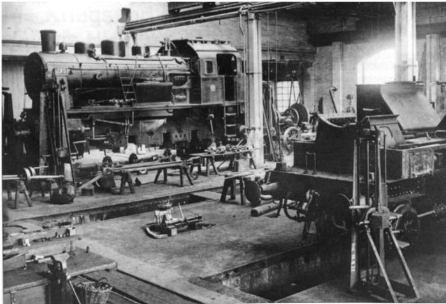
Vom Ausbesserungswerk in Nietleben gibt es leider sehr wenig Bilddokumente. Umso erfreulicher das Bild von Lok 185 auf Hebeböcken in dieser Werkstatt. Im Vordergrund das Fahrgestell und der Rahmen einer 1'Ch2t-ELNA Aufnahme: Sammlung H.-D. Rammel
