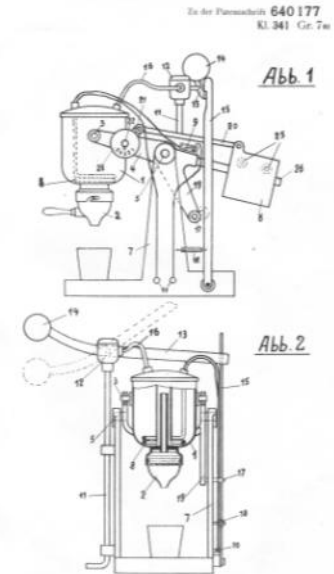
Entwurf Elektrische Brühvorrichtung für Kaffee u.a. (Patent 1936)
